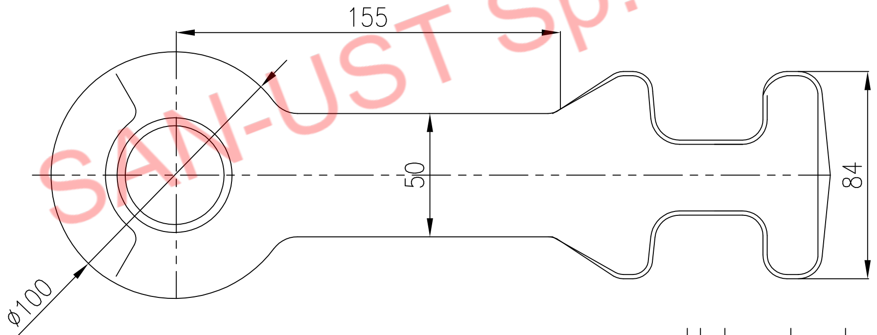
Ucho dyszla D43.19.07
